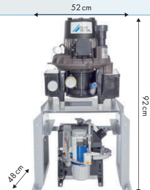
VSA 600
