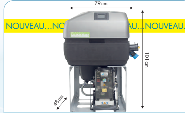
TYSCOR VSA 4
